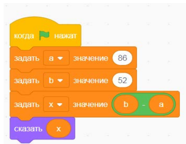
Рис. 118. Вид программы
