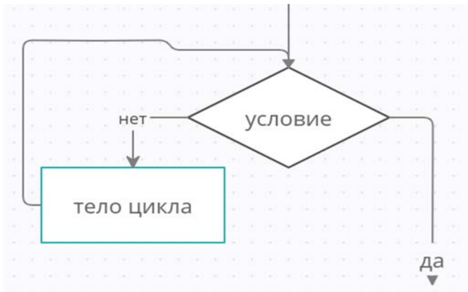
Рис. 127. Блок-схема цикла
